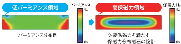
IPMモーター用磁石のパーミアンス分布例
