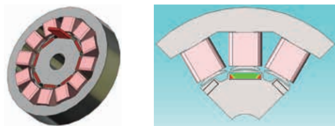
IPMモーター用磁石のパーミアンス分布例
