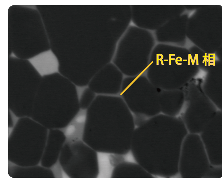
(反射電子組成像)
