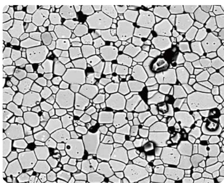
(粒界相エッチング後の組織)
