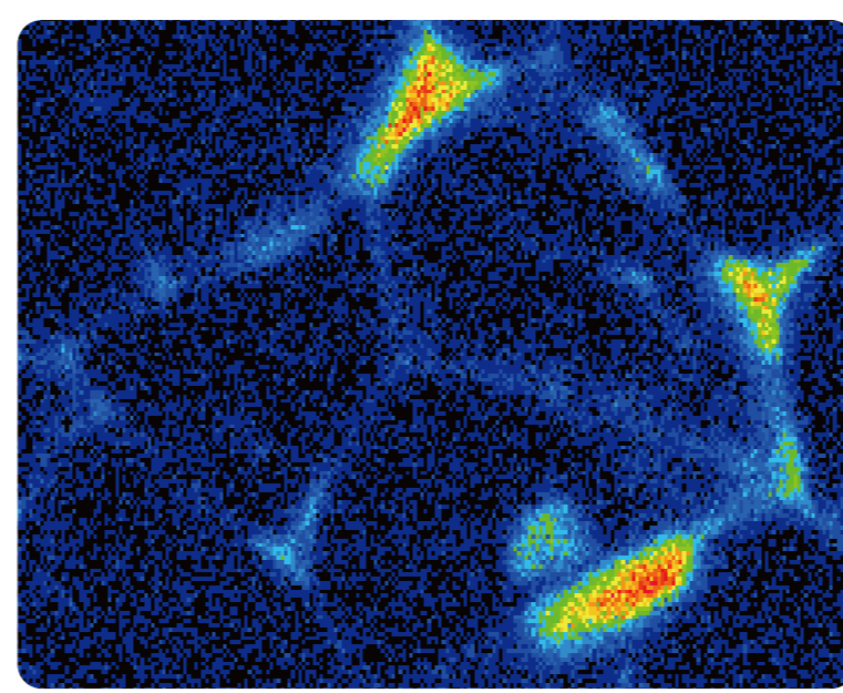
(重希土類元素の組織内分布)
